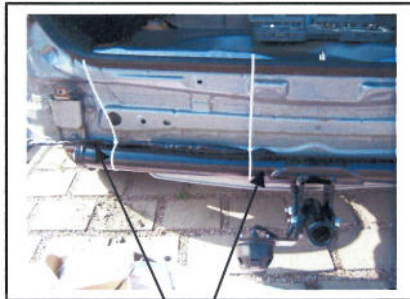
Kabelführung zu Steckdose entlang Aufhängung
