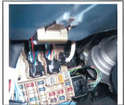
8pol. Relaisstecker abstecken
